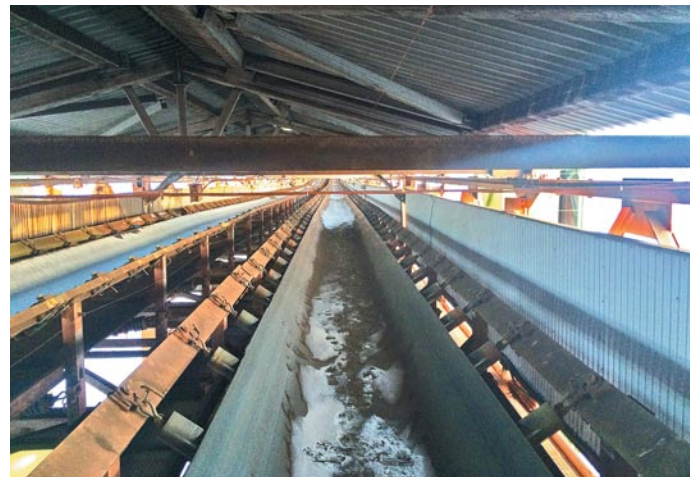
Красноярский край. АО «Разрез Березовский». Подвес оптоволоконного ЧЭ над лентой конвейера.
